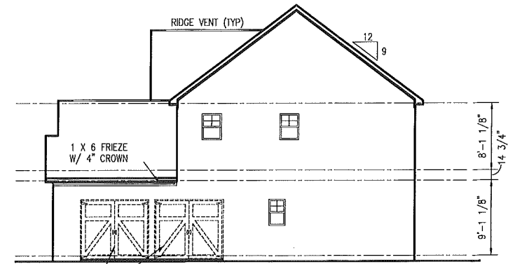
RIGHT ELEVATION
