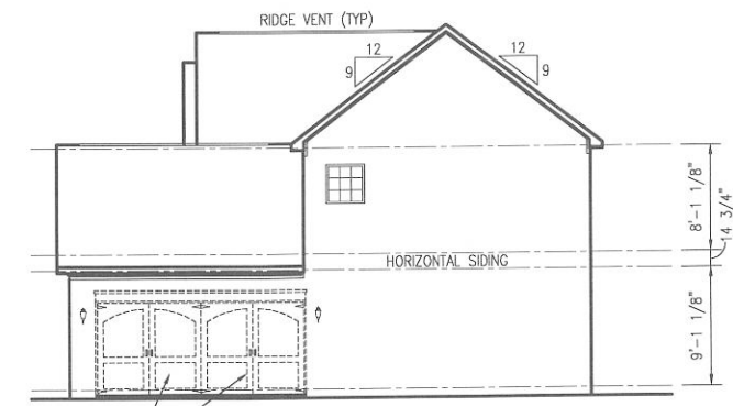
RIGHT ELEVATION
