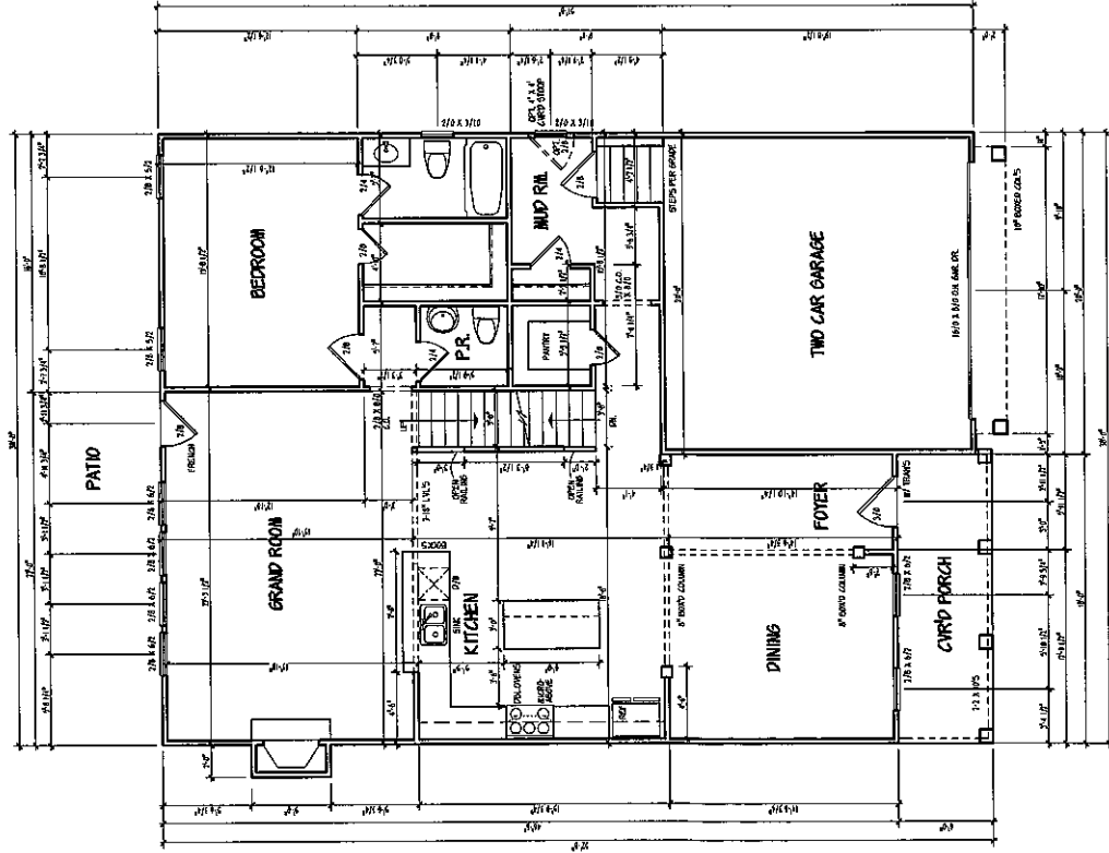
MAIN LEVEL PLAN SCALE: 1/8" = 1'-0"
